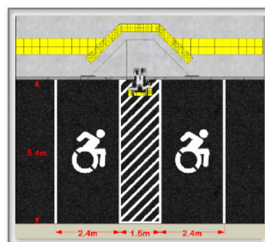
NBC B-3.5.a) Dimensions
